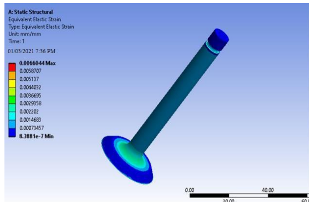
Figure12:StrainofvalveusingAl+Sic(30%)
