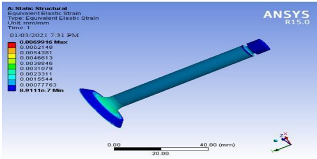
Figure9:Fig:StrainofvalveusingAl+Sic(20%)
